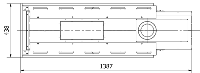
B-B (1 : 10)
