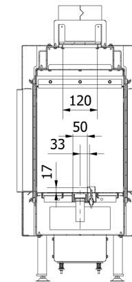
A-A (1 : 10)
